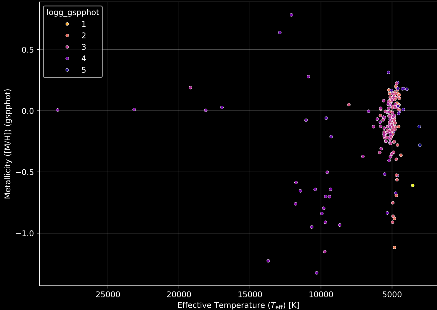
APOGEE DR17 Field: [191+04] Stellar Population Parameters (n= 204)
